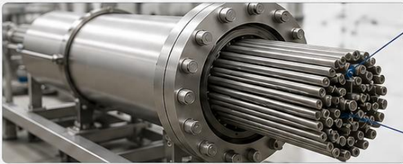
MEMBRANE MODULE
